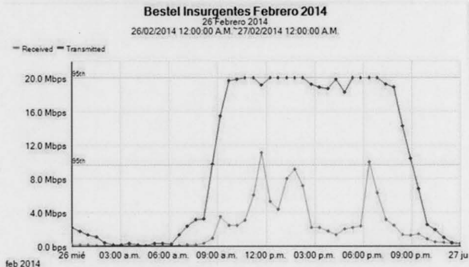
Ilustración 3 Enlace Internet, Operbes - IFAI Febrero de 2014
