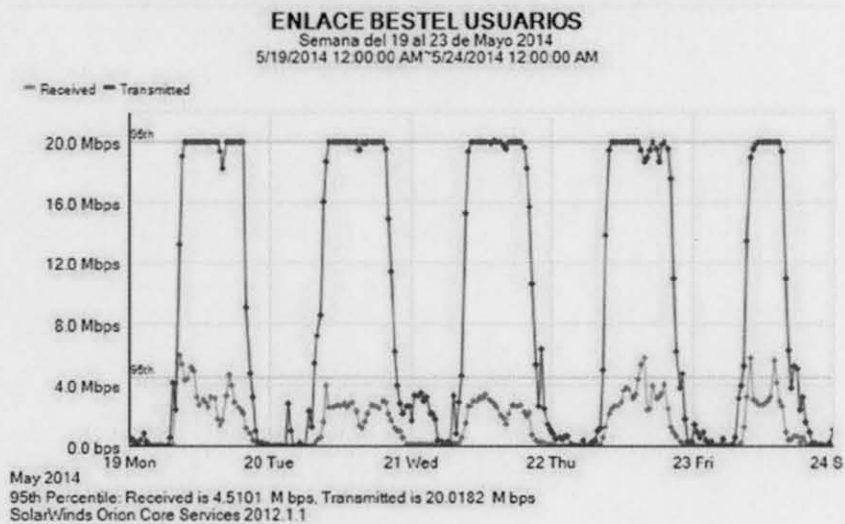
Ilustración 1 Enlace Internet, BESTEL- IFAI Mayo de 2014
